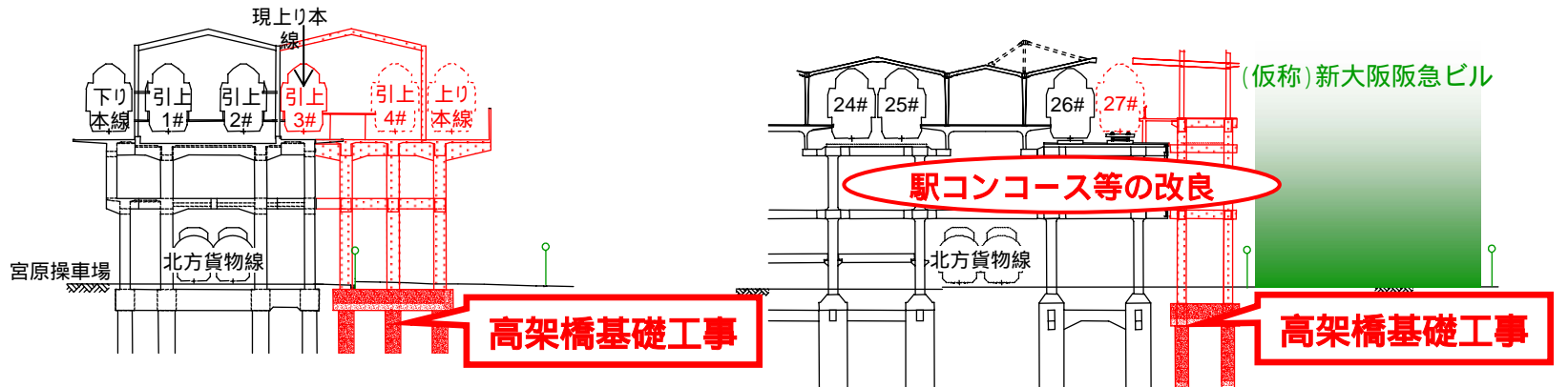
断面図【引上線部】
