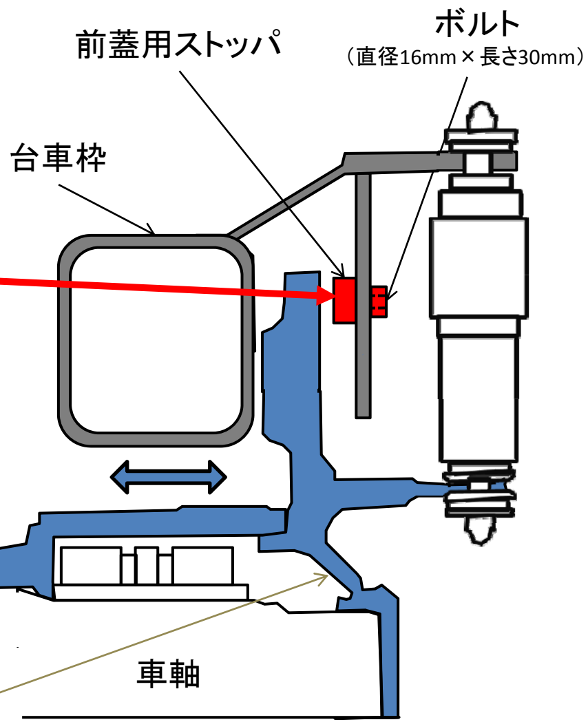
＜断面図A-B＞
