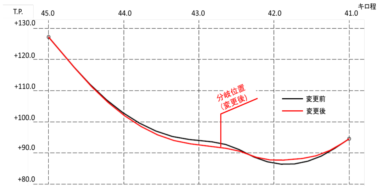
縦断面図
