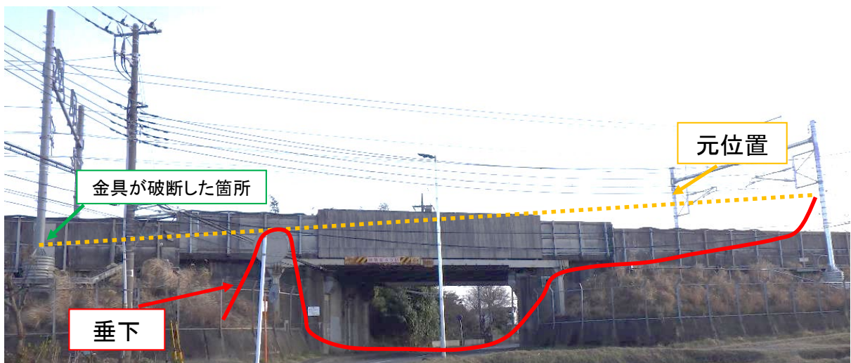
ワイヤー垂下の状況
